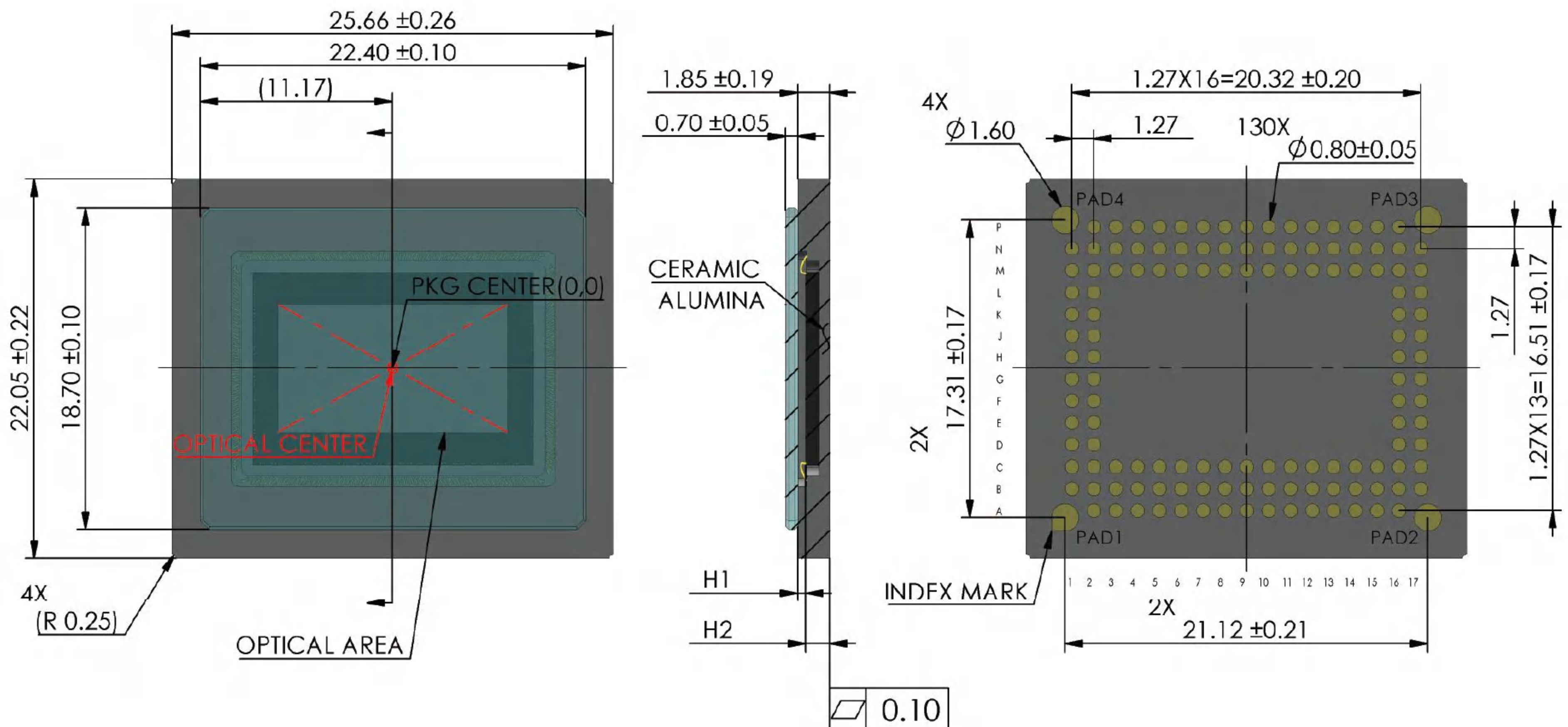
封装图示
